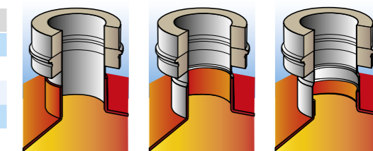
Adaptador caldera interior, Adaptador caldera exterior, Adaptador caldera antihollín
