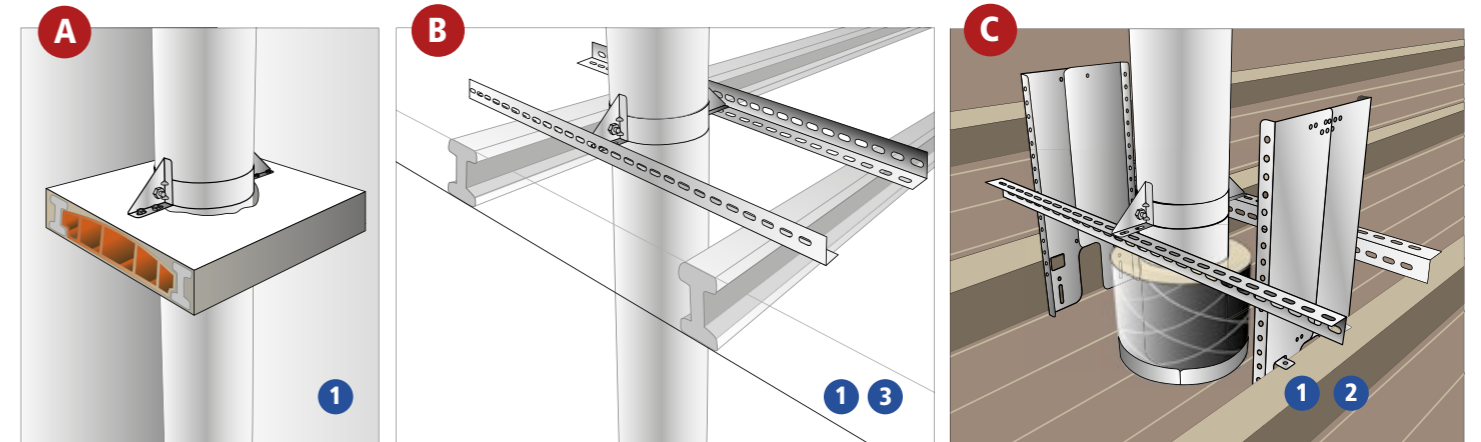
Abrazadera forjado
