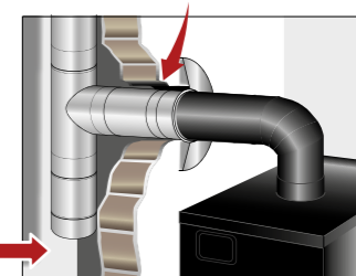
Paso mural
