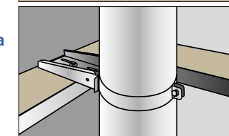
Abrazadera forjado reforzada
