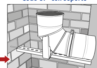
Codo 87° con soporte
