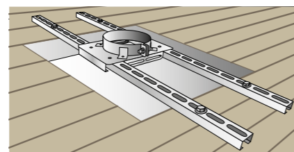
Kit fijación soporte mural universal
