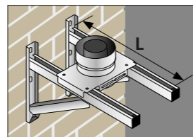
Escuadra reforzada con soporte mural
