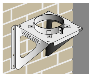
Escuadra con soporte mural universal
