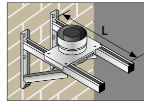
Escuadra reforzada con soporte mural
