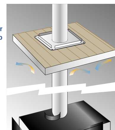
Distanciador de fuego
