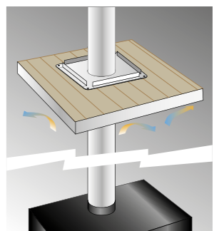
Distanciador de fuego
