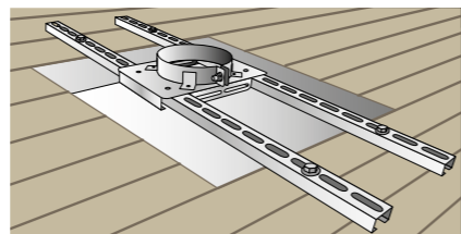
Kit fijación soporte mural universal
