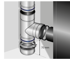
Te base
