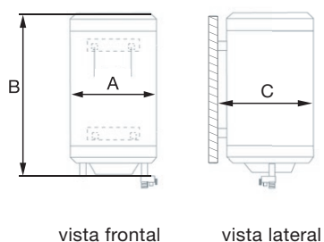
Esquema de medidas termo digital DELTA Ultimate
