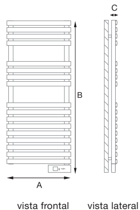
Esquema de medidas secatoallas DELTA Ultimate
