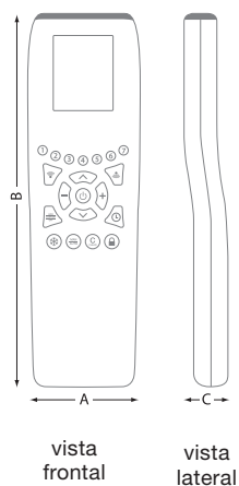
Esquema de medidas mando AIR Control
