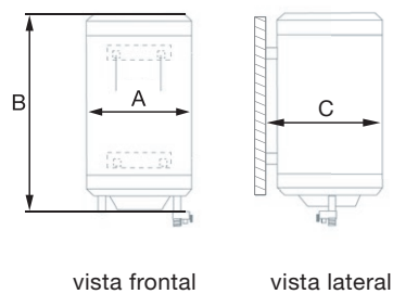
Esquema de medidas termo digital SYGMA
