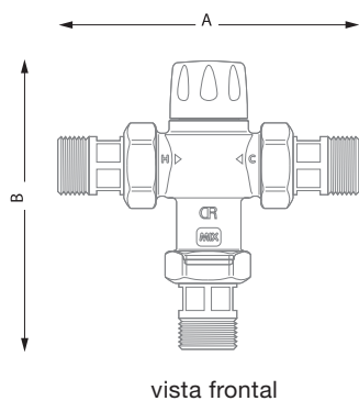
Esquema de medidas Kit ahorro energético para termos
