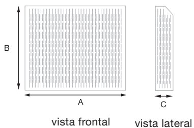
Esquema de medidas rejilla protectora para radiadores KYROS y SYGMA
