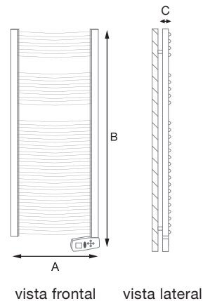
Esquema de medidas secatoallas SYGMA
