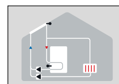
Solar con refrigeración 2 (refrigeración del colector)
