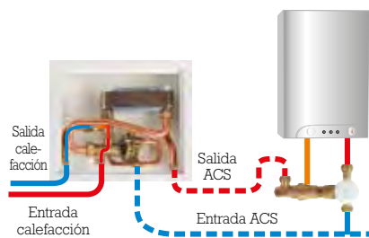
Si no hay demanda de ACS:
