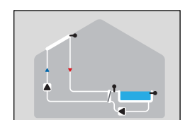
Solar con piscina e intercambiador de calor
