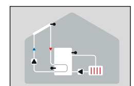
Solar con refrigeración 3 (refrigeración del almacenamiento)
