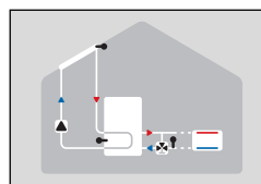
Solar con circuito calefactor
