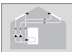
Solar con dos superficies colectoras y dos bombas
