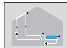
V3 y V4: solar con intercambiador de calor (sensor en el segundo circuito) y piscina
