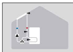
Solar con bypass
