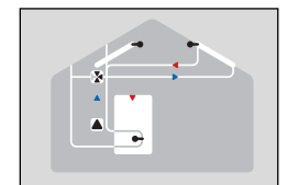
Solar con dos superficies colectoras
