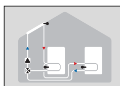
Solar con dos almacenamiento y una válvula
