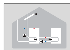
Solar con transmisor de almacenamiento
