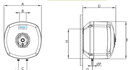
EV-10 / EV-15 / EV-30 Sobre fregadero
