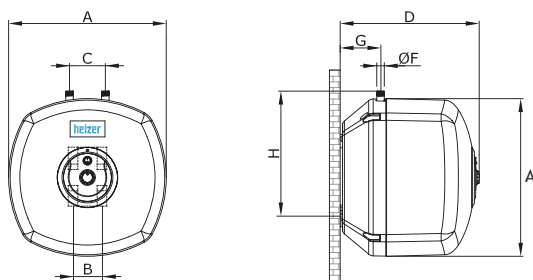
EV-10 / EV-15 Bajo fregadero
