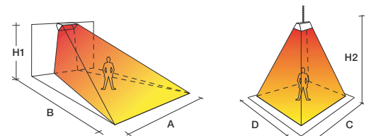
Esquema de Instalación y área radiada
