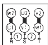
Conexión de motores Estrella/triángulo
